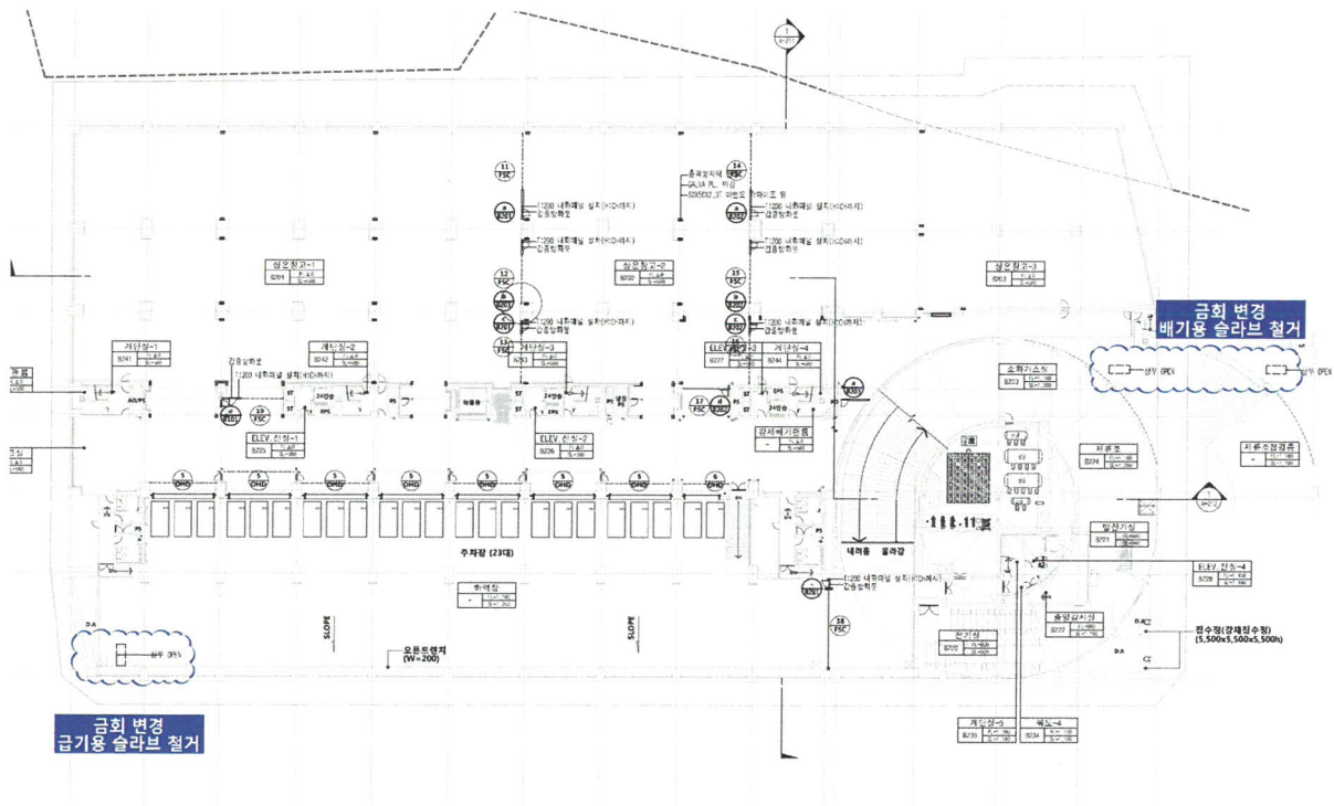
1) 평면도_지하 2층
